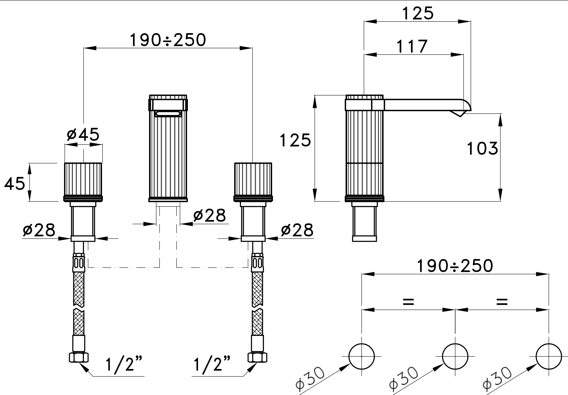
schema fori - modèle de trou hole pattern - patròn de agujero
