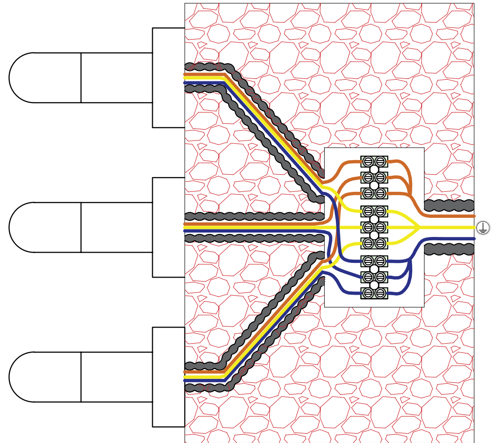
Schema när extern strömbrytare ska användas
